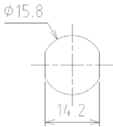
取付穴寸法
