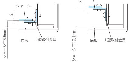
取付図
