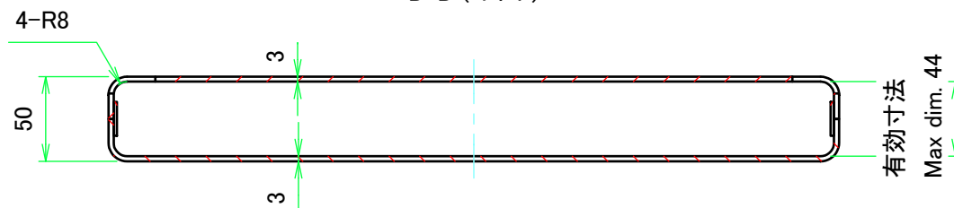
D-D (1:4)
