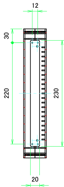
A-A (1:4)
