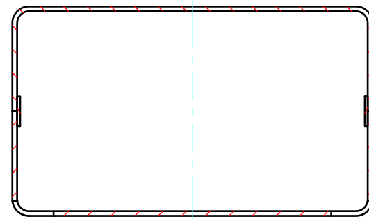
C-C (1:3.5)
