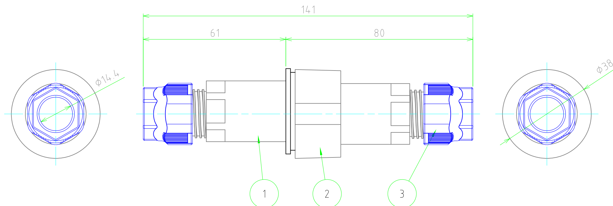
展開図
