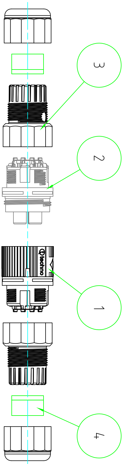
展開図
