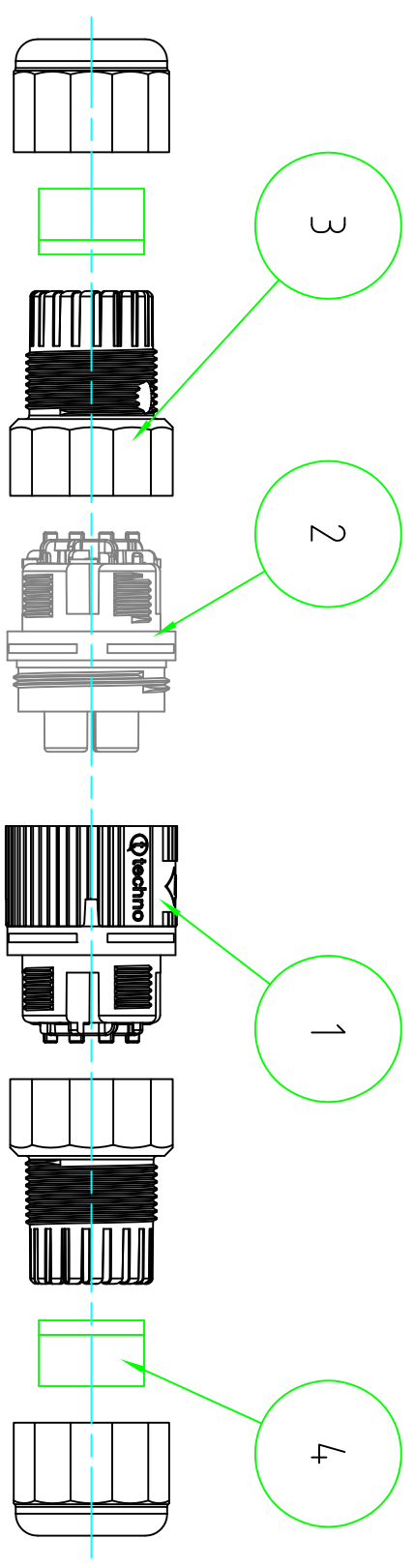
展開図
