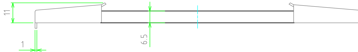
取付穴寸法図
