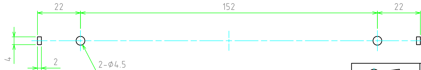
取付穴寸法図
