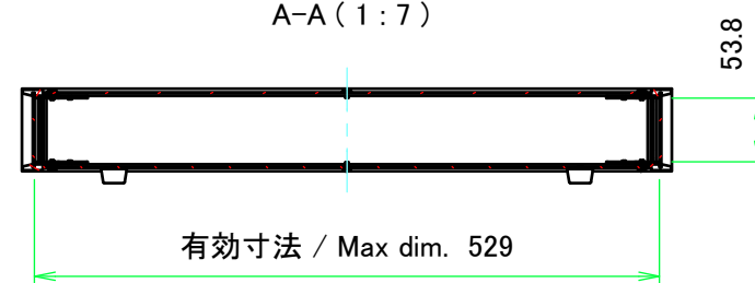
A-A (1:7)
