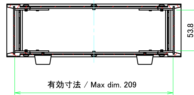
A-A (1:3)
