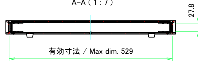
A-A (1:7)
