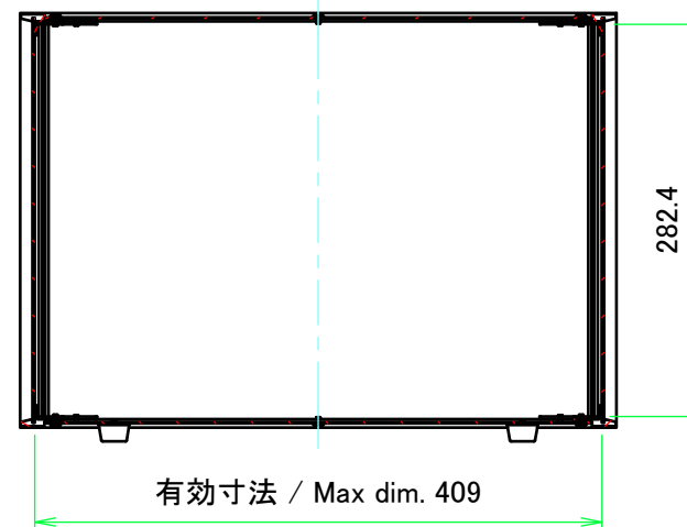
A-A (1:6)
