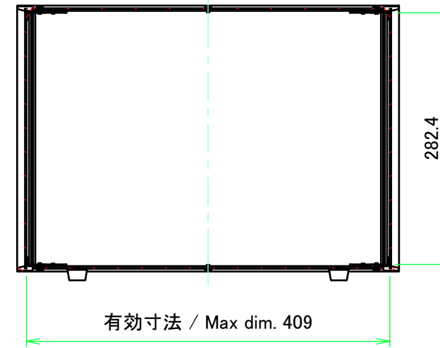
A-A (1:6)
