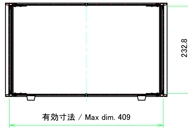
A-A (1:6)
