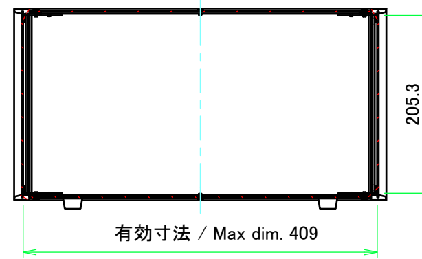
A-A (1:6)
