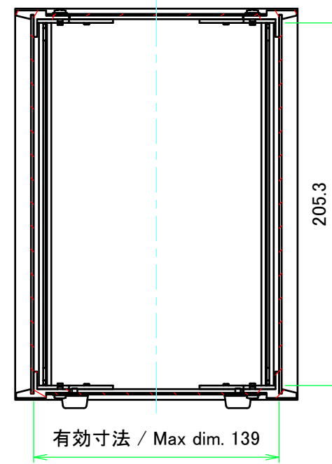
A-A (1:3)
