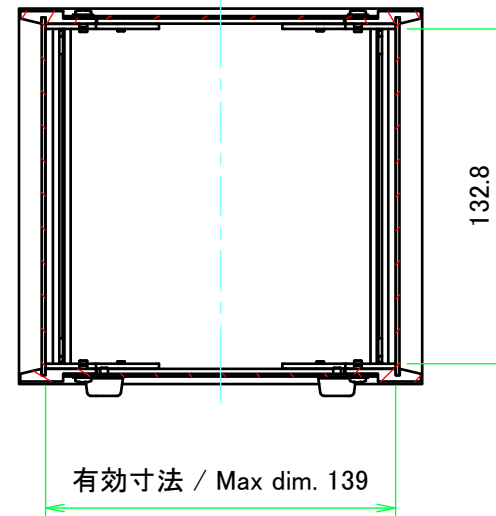
A-A (1:3)
