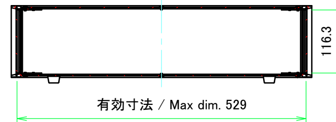
A-A (1:7)
