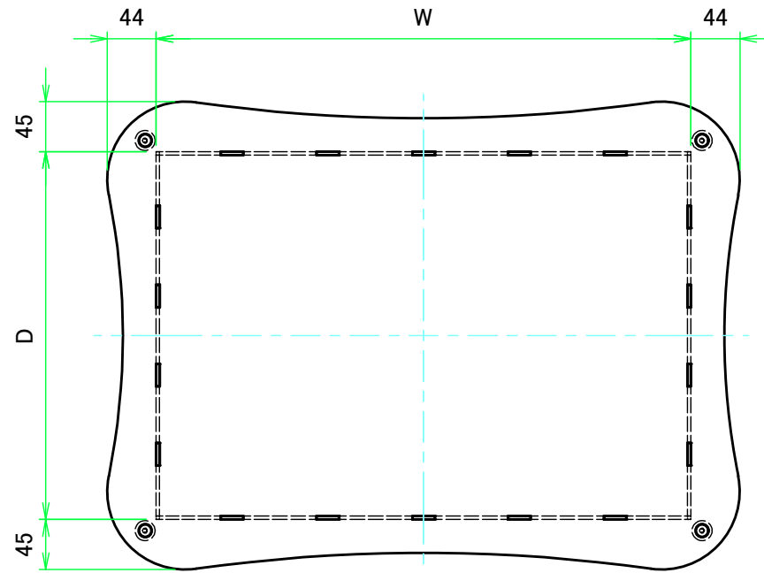
上カバー / Top cover
