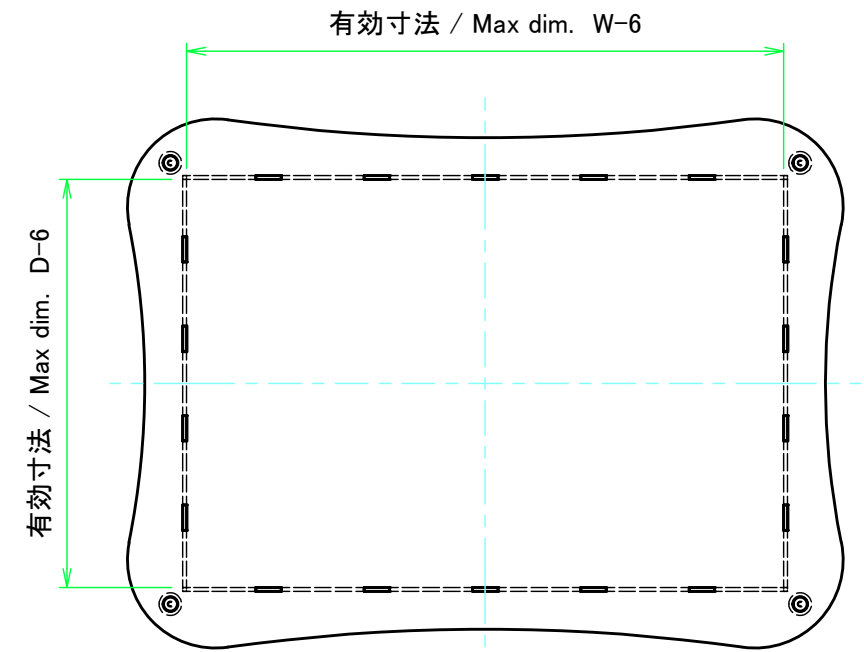
下カバー / Bottom cover
