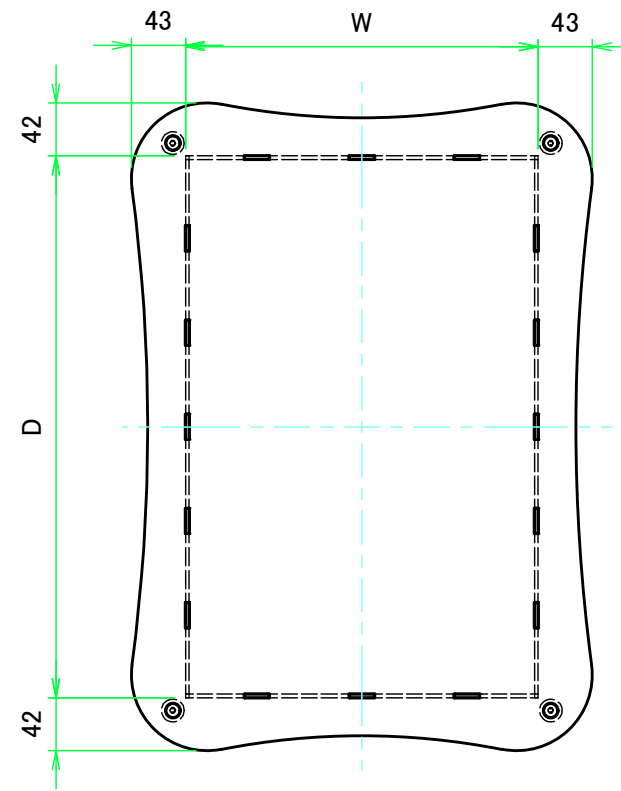
Wパネル1 / W panel 1
