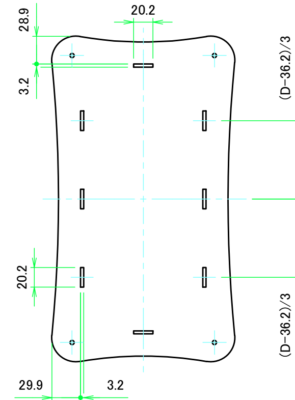
上カバー裏面 / Top cover Backside
