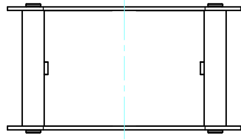
上カバー / Top cover
