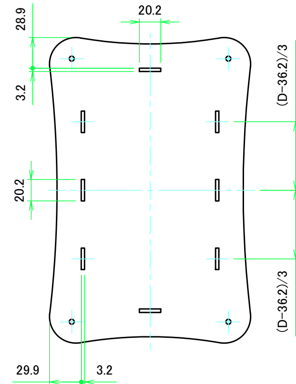
上カバー裏面 / Top cover Backside
