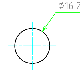
取付穴寸法 / Mounting hole dimensions
