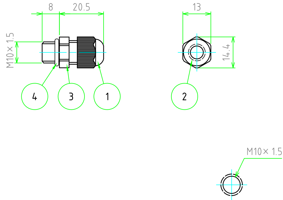
取付穴寸法 / Mounting hole dimensions
