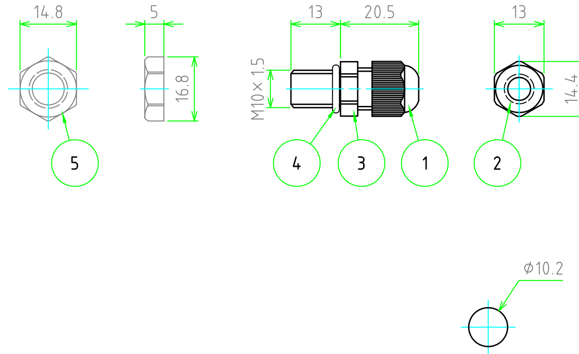
取付穴寸法 / Mounting hole dimensions
