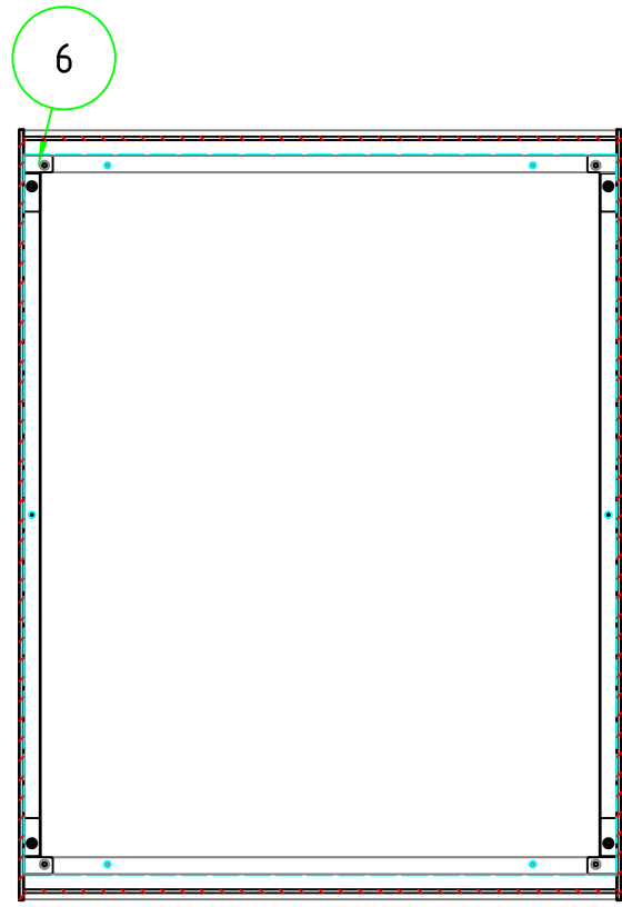
C-C 断面図
