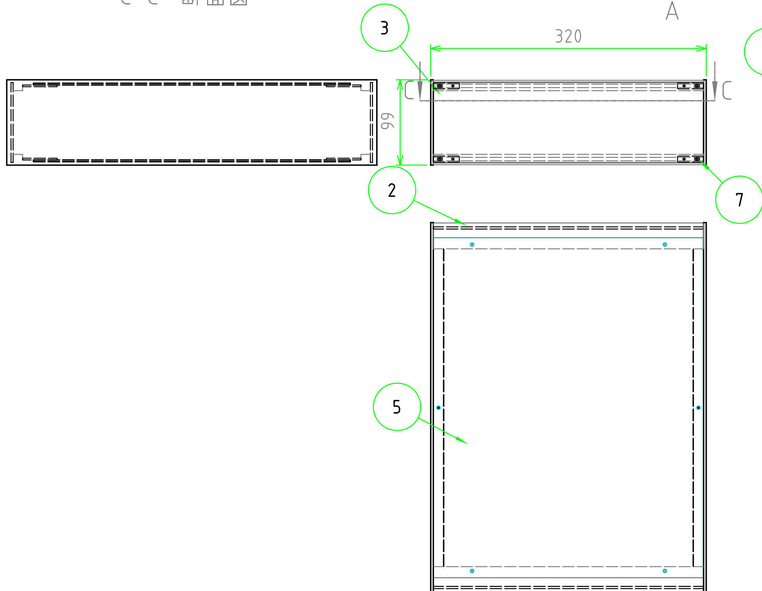
C-C 断面図
