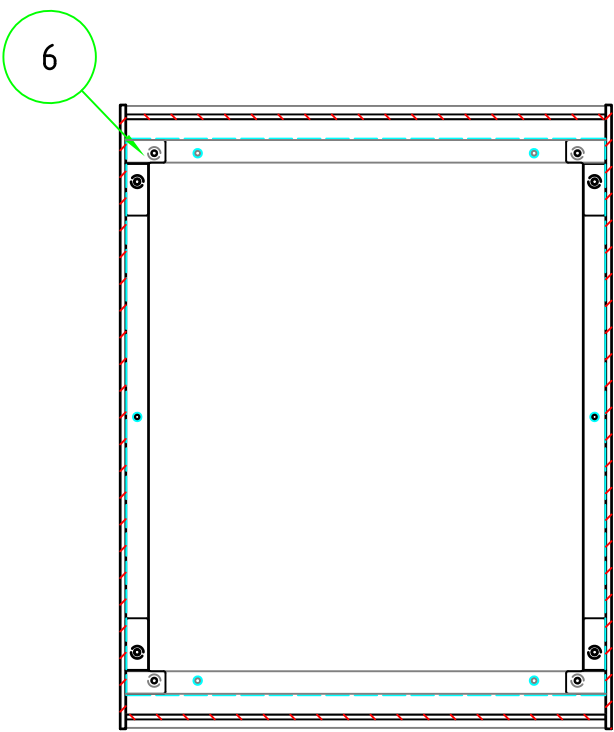
C-C 断面図
