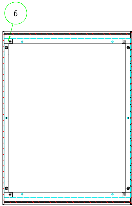
C-C 断面図
