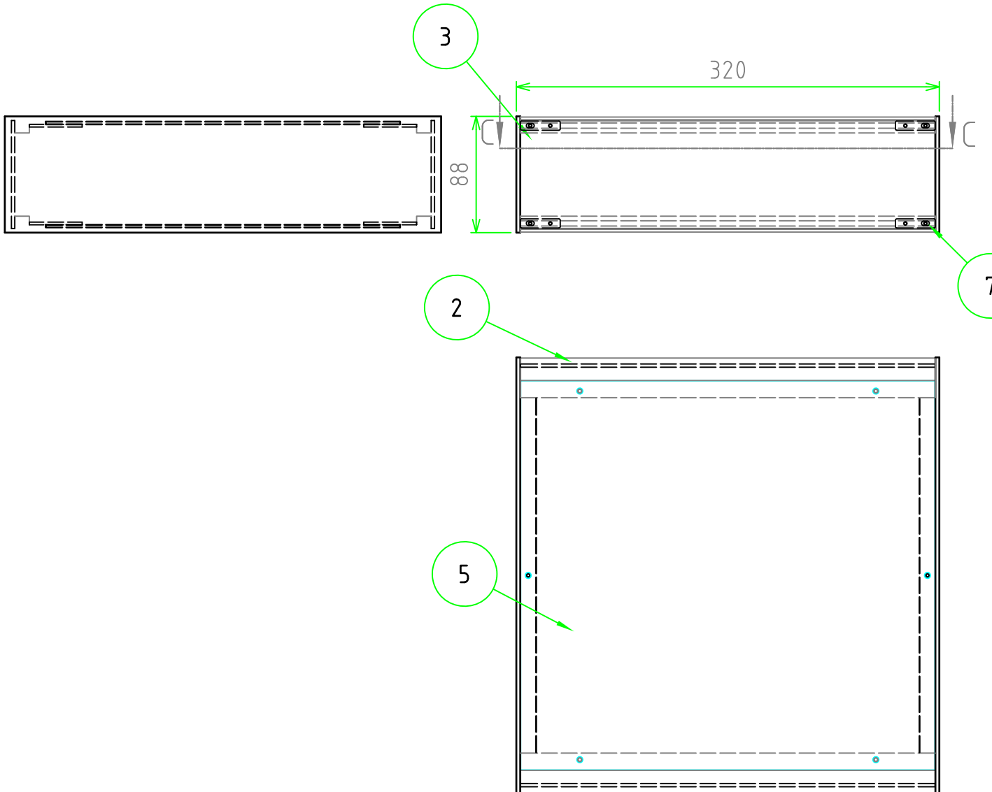
C-C 断面図
