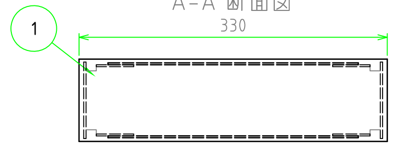
A-A 断面図
