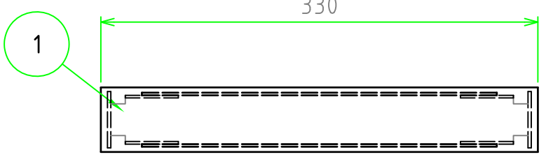
A-A 断面図
