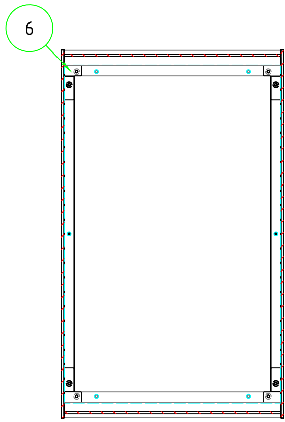
C-C 断面図
