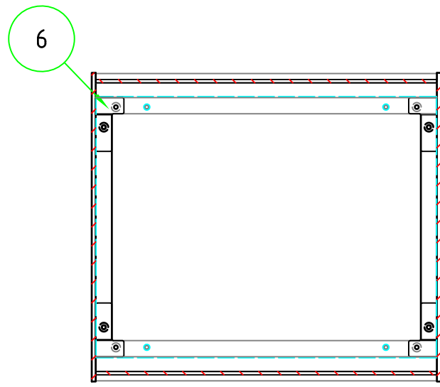
C-C 断面図
