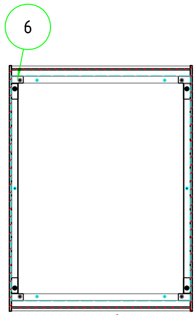
C-C 断面図
