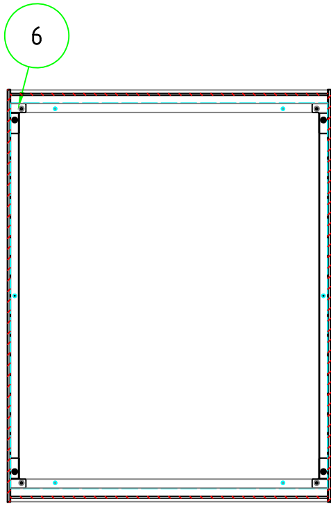
C-C 断面図
