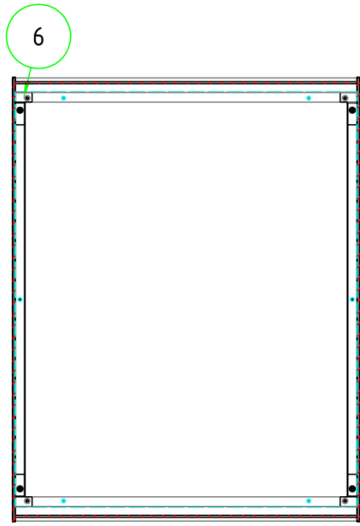
C-C 断面図
