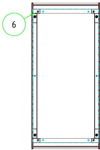
C-C 断面図
