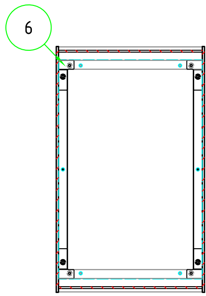
C-C 断面図
