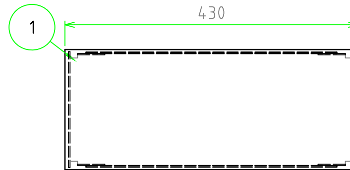
A-A 断面図
