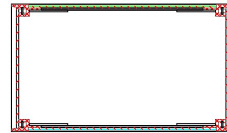
A-A 断面図
