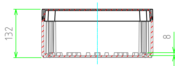
D-D
