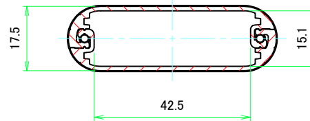
A-A (1:1)
