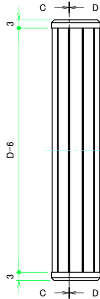
D-D (1:1)
