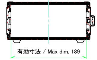
リアフレーム2 / Rear frame2
