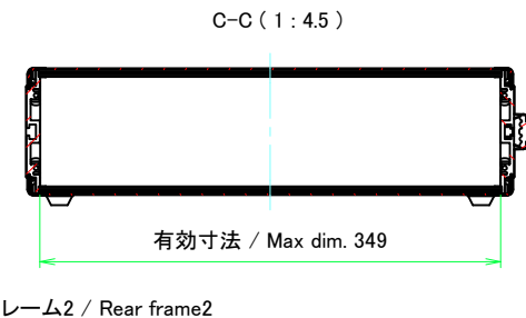
リアフレーム2 / Rear frame2
