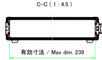
リアフレーム2 / Rear frame2
