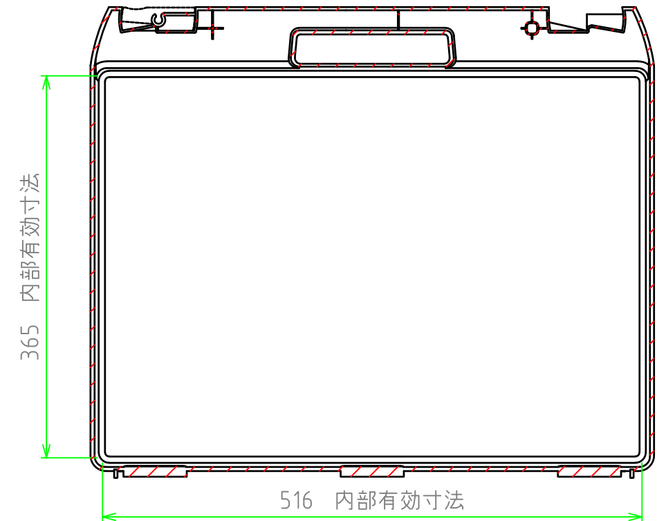
B-B 断面図
