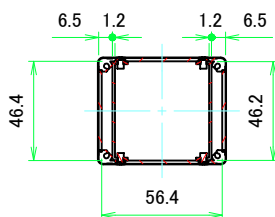
A-A (1:2.5)
