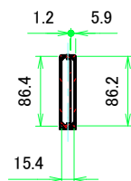
A-A (1:6)
