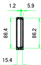
A-A (1:4.5)
